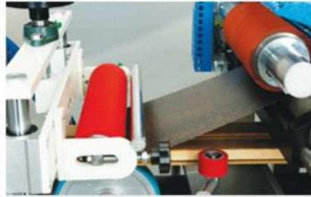
Tutkallanmış Malzemeyi Kesişim Noktasında Hizalayan Basık Merdanesi The Pres Rolls Is Aling Glued Material in Intersection Point
